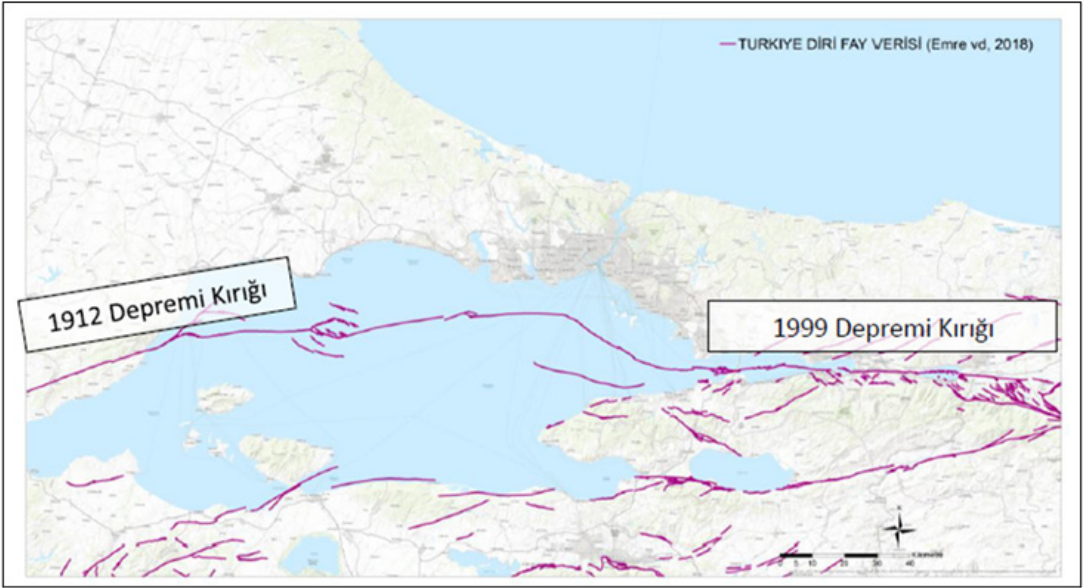
Şekil 4-2: Marmara Bölgesi Diri Fay Verisi (Emre ve dig., 2018 verisi ile çizilmiştir.)
