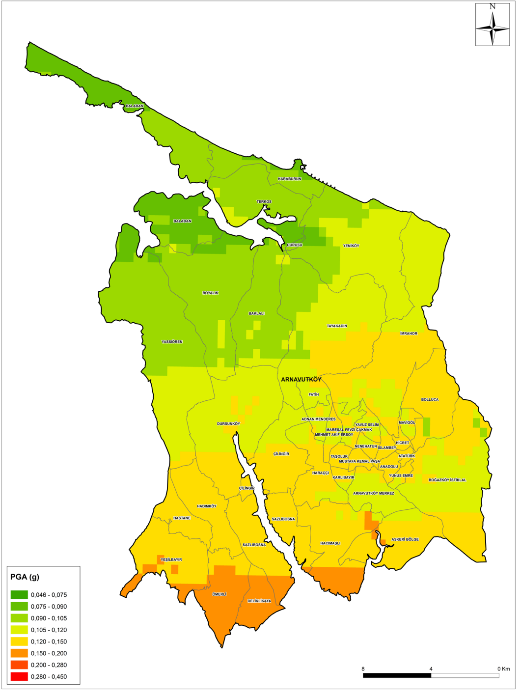
Şekil 4-4: Senaryo Depremi İçin Elde Edilen Arnavutköy İlçesi Zemin Bağımlı Medyan En Büyük Yer İvmesi (PGA) Dağılımı
