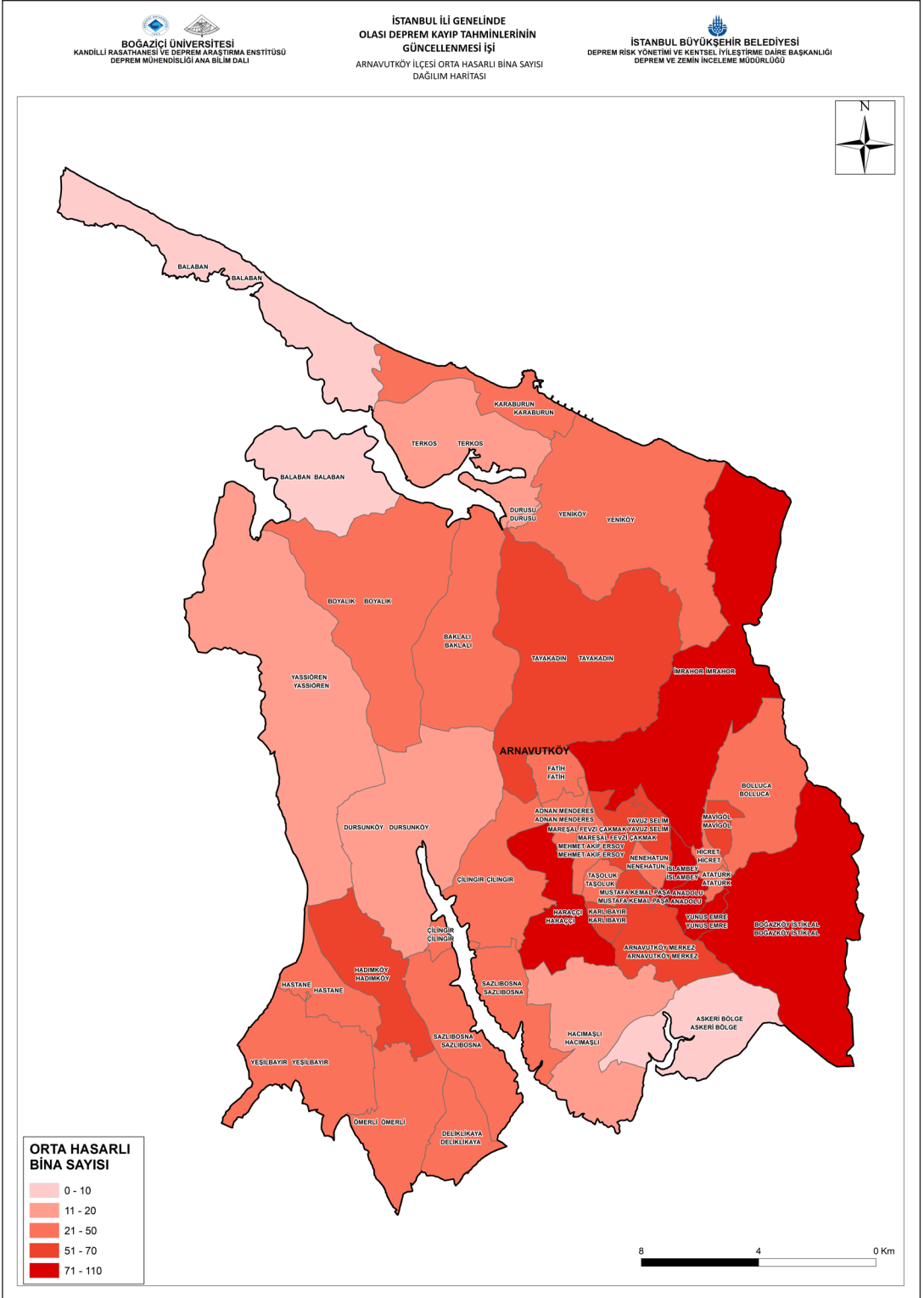
Şekil 5-4: Mw=7.5 Senaryo Depremi İçin Arnavutköy İlçesi Tahmini Orta Hasarlı Bina Sayısı Dağılım Haritası
