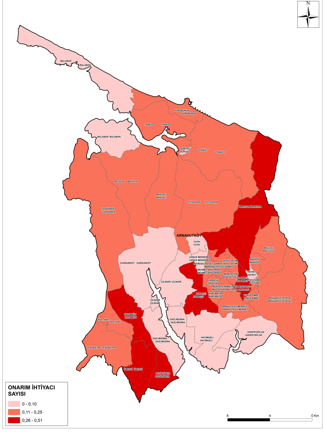
Şekil 5-10: Mw=7.5 Senaryo Depremi İçin Arnavutköy İlçesi Doğal Gaz Şebekesi Boru Hatları Tahmini Onarım İhtiyacı Dağılım Haritası
