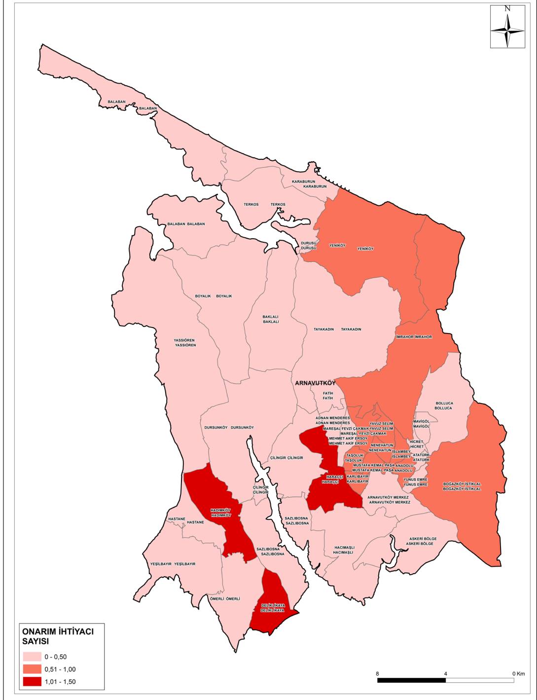
Şekil 5-11: Mw=7.5 Senaryo Depremi İçin Arnavutköy İlçesi İSKİ Atık Su Boru Hatları Tahmini Onarım İhtiyacı Dağılım Haritası
