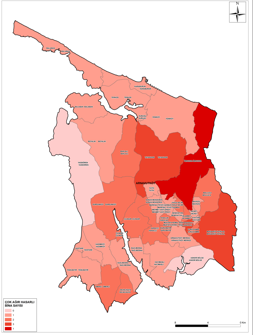
Şekil 5-2: Mw=7.5 Senaryo Depremi İçin Arnavutköy İlçesi Tahmini Çok Ağır Hasarlı Bina Sayısı Dağılım Haritası
