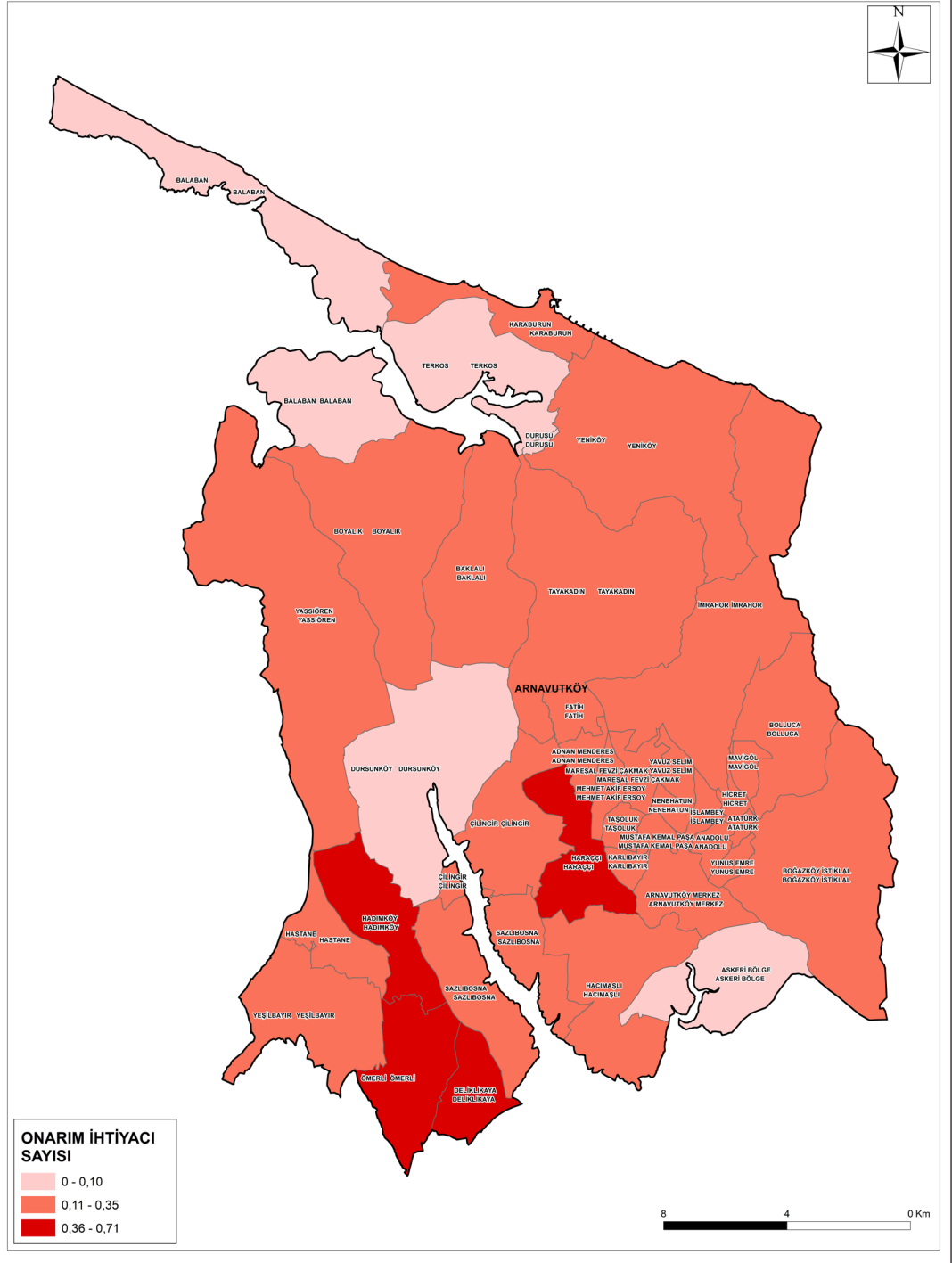
Şekil 5-12: Mw=7.5 Senaryo Depremi İçin Arnavutköy İlçesi İSKİ İçme Suyu Boru Hatları Tahmini Onarım İhtiyacı Dağılım Haritası
