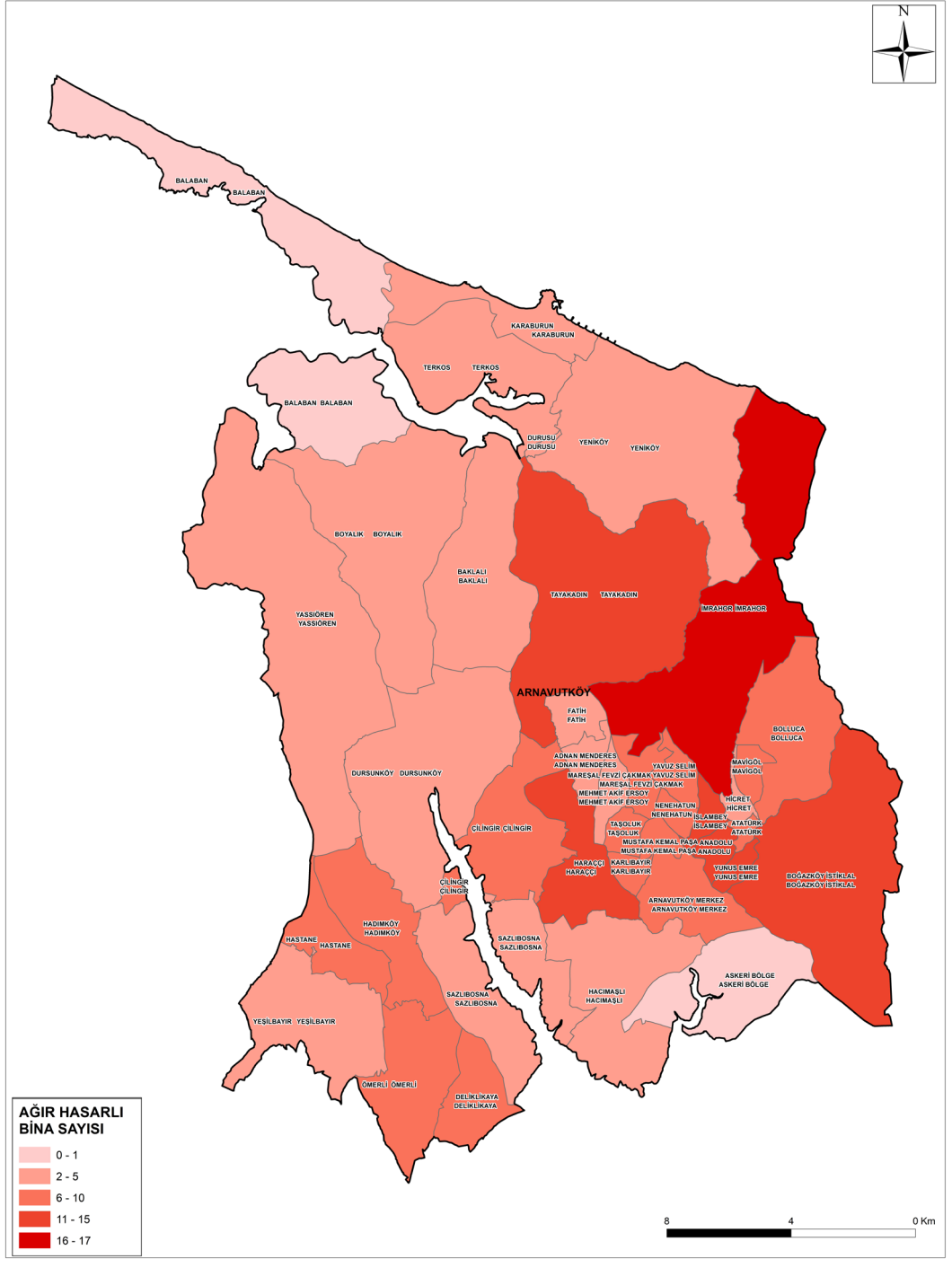
Şekil 5-3: Mw=7.5 Senaryo Depremi İçin Arnavutköy İlçesi Tahmini Ağır Hasarlı Bina Sayısı Dağılım Haritası
