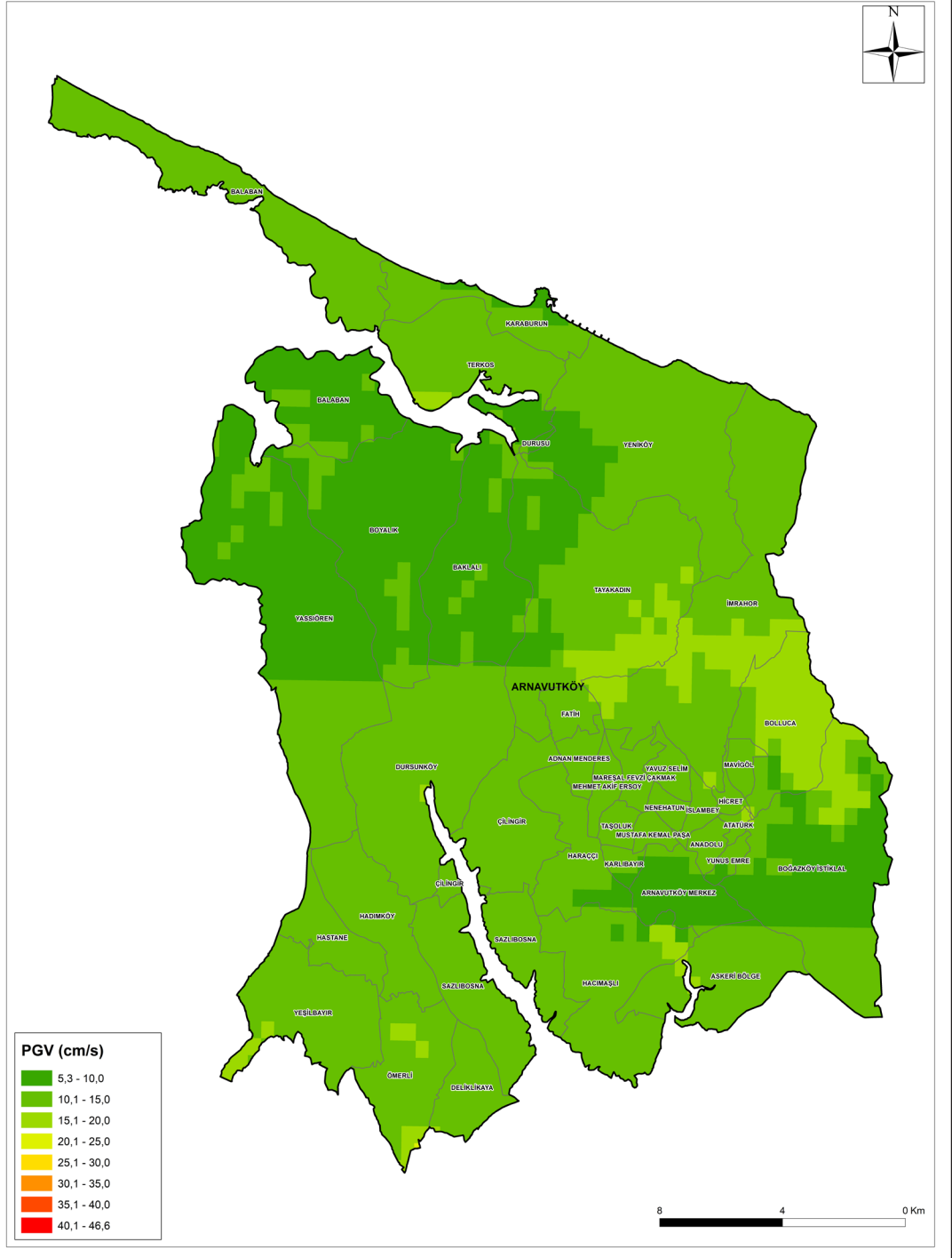
Şekil 4-5: Senaryo Depremi İçin Elde Edilen Arnavutköy İlçesi Zemin Bağımlı Medyan En Büyük Yer Hızı (PGV) Dağılımı
