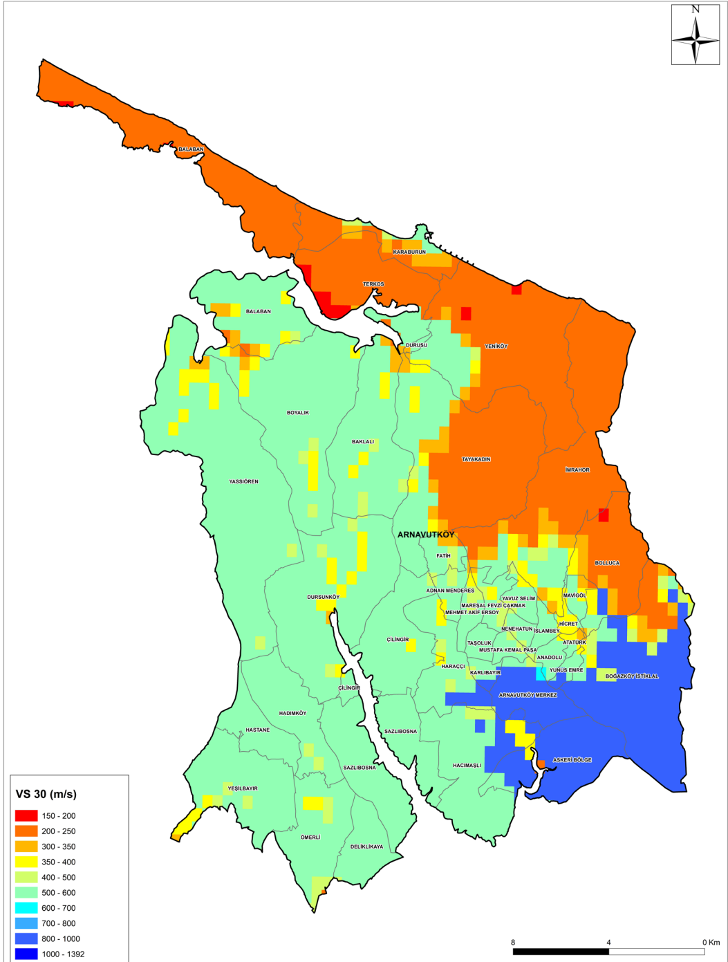
Şekil 4-1: Arnavutköy İlçesi V_{s30} Dağılımı
