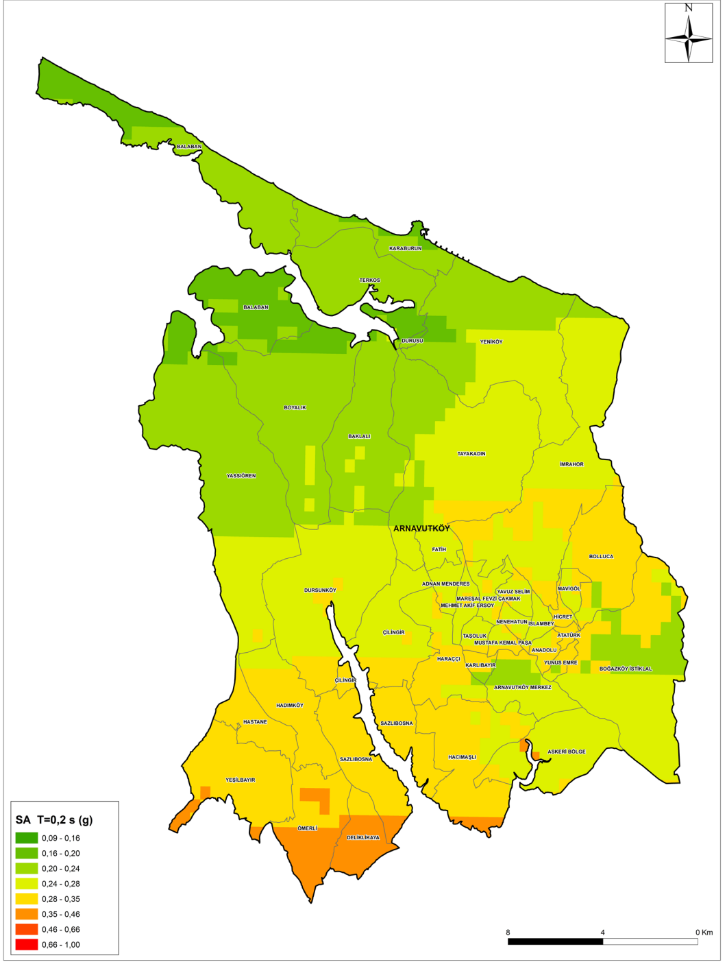
Şekil 4-6: Senaryo Depremi İçin Elde Edilen Arnavutköy İlçesi Zemin Bağımlı T=0.2 s İçin Spektral İvme Dağılımı
