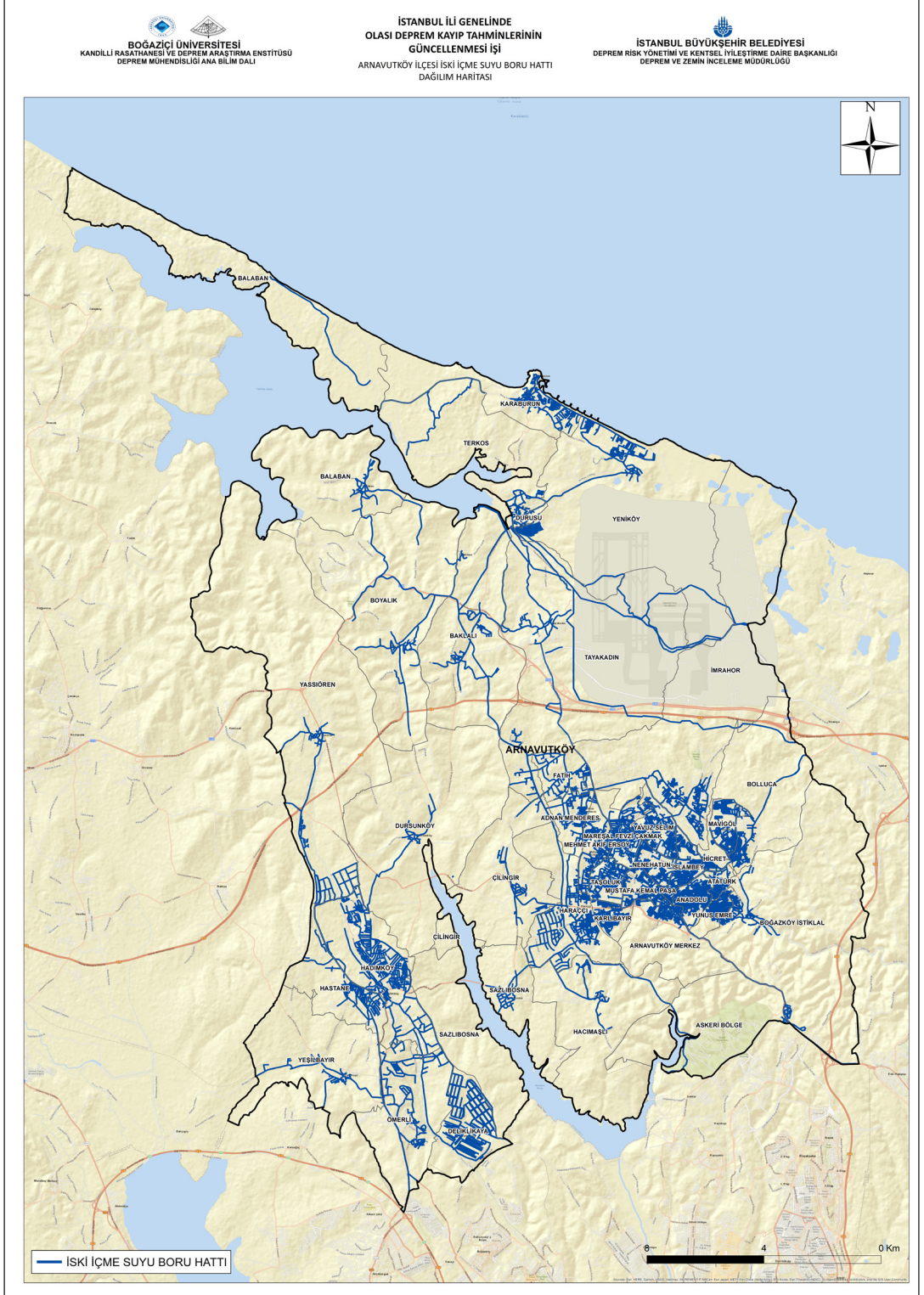
Şekil 3-10: Arnavutköy İlçesi İSKİ İçme Suyu Boru Hattı Dağılımları
