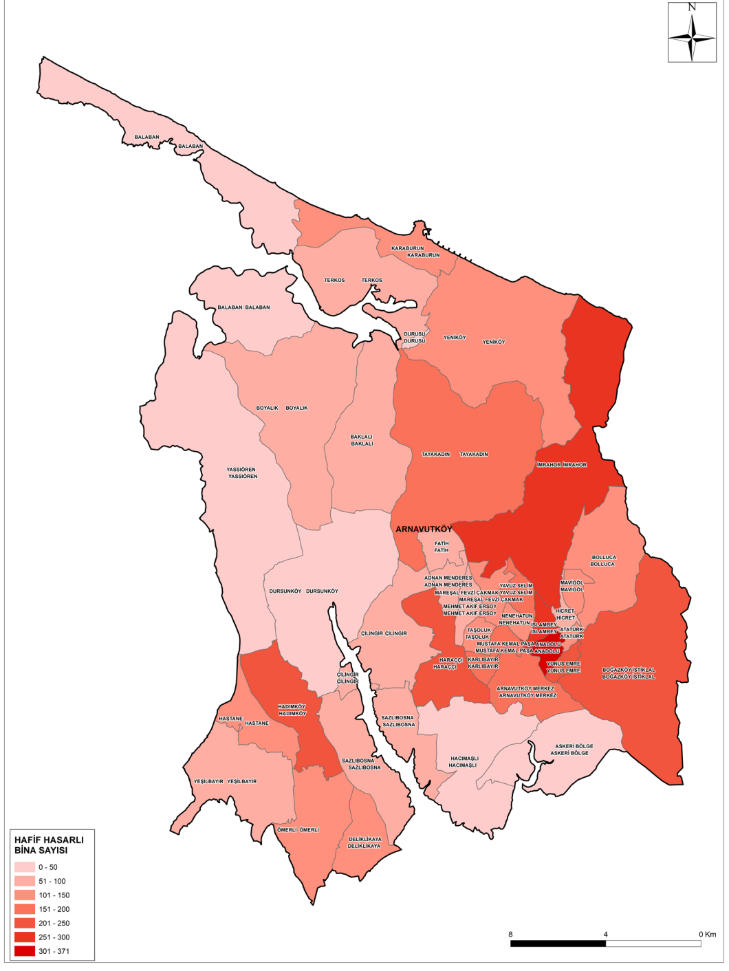
Şekil 5-5: Mw=7.5 Senaryo Depremi İçin Arnavutköy İlçesi Tahmini Hafif Hasarlı Bina Sayısı Dağılım Haritası
