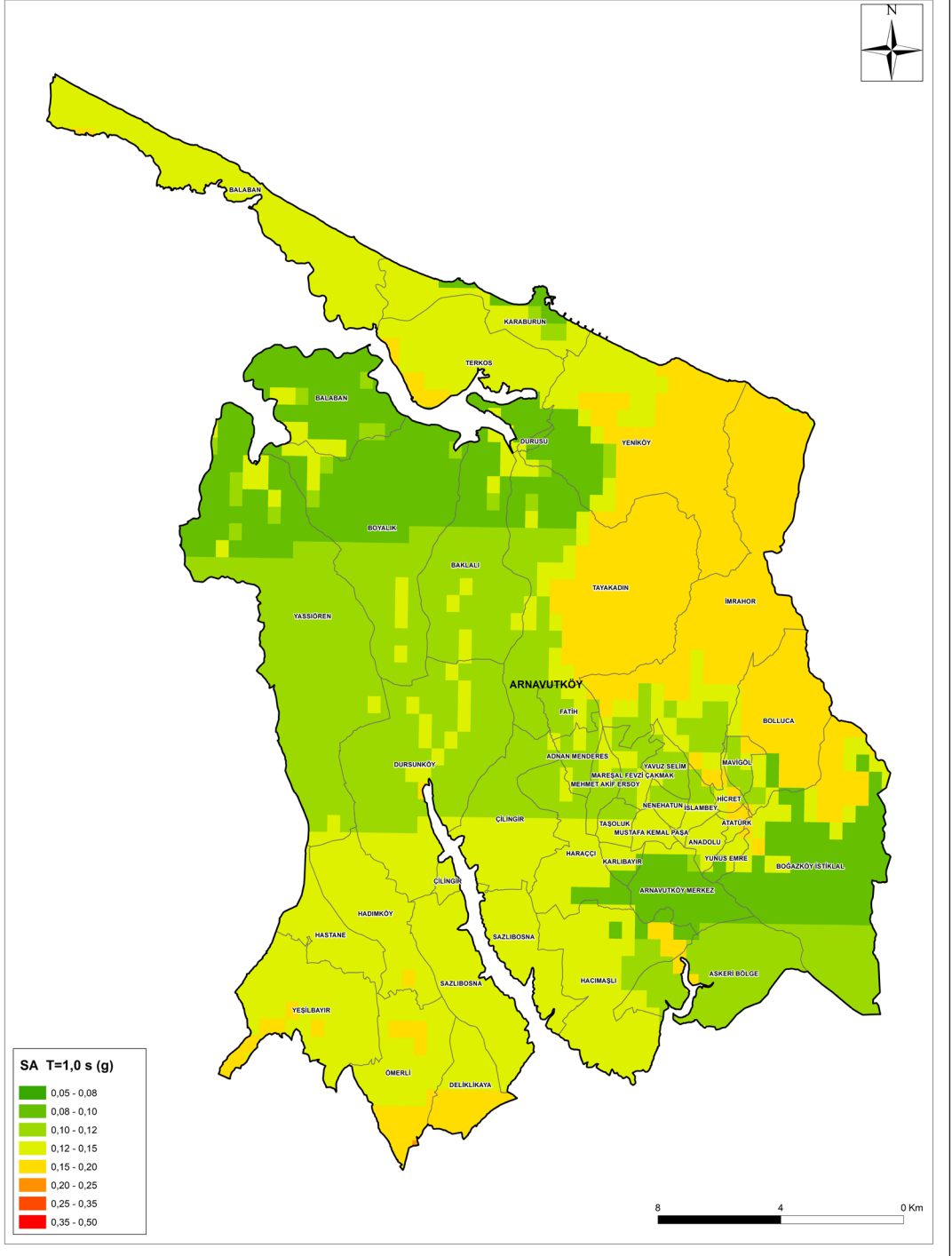
Şekil 4-7: Senaryo Depremi İçin Elde Edilen Arnavutköy İlçesi Zemin Bağımlı T=1.0s için Spektral İvme Dağılımı
