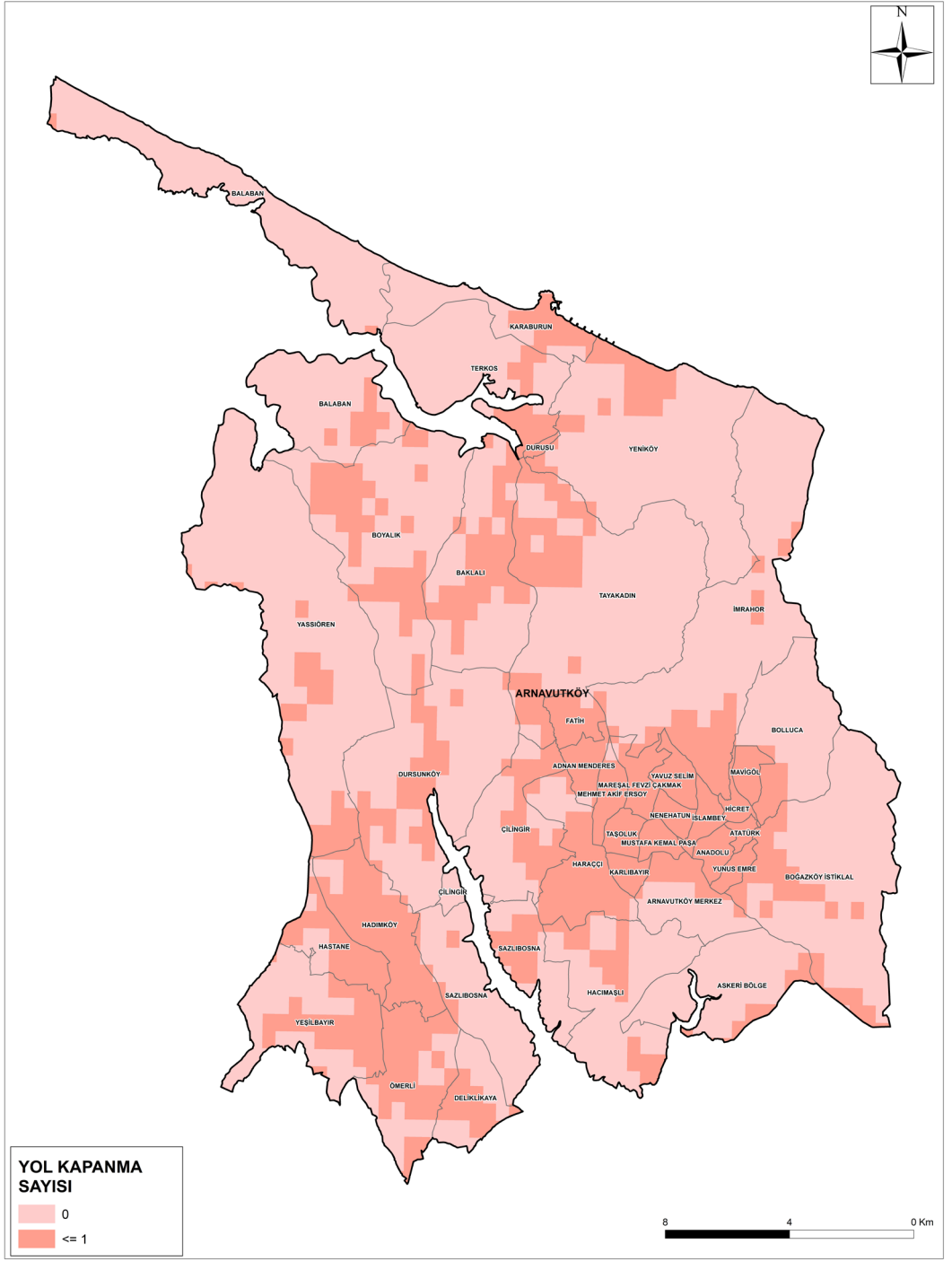
Şekil 5-13: Mw=7.5 Senaryo Depremi için Arnavutköy İlçesi Yol Kapanma Dağılım Haritası
